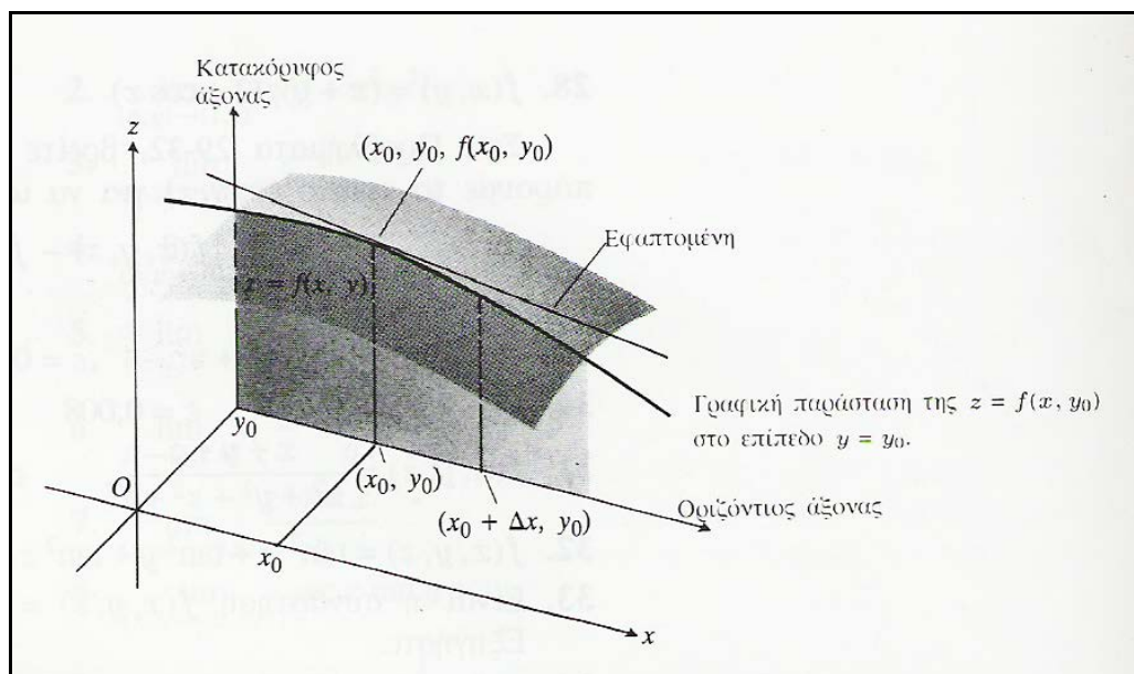
Σχήμα 2. Γραφική παράσταση της z = f(x, y) στο επίπεδο y = y_0 .
