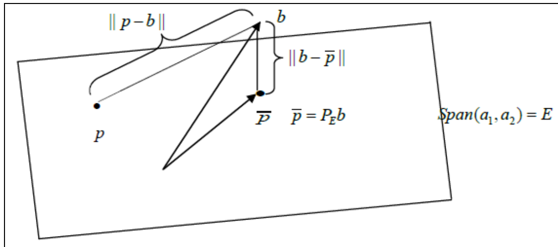
Σχήμα 1. Απεικόνιση της προβολής \bar{p} του b στο επίπεδο Span(a_1, a_2) .
